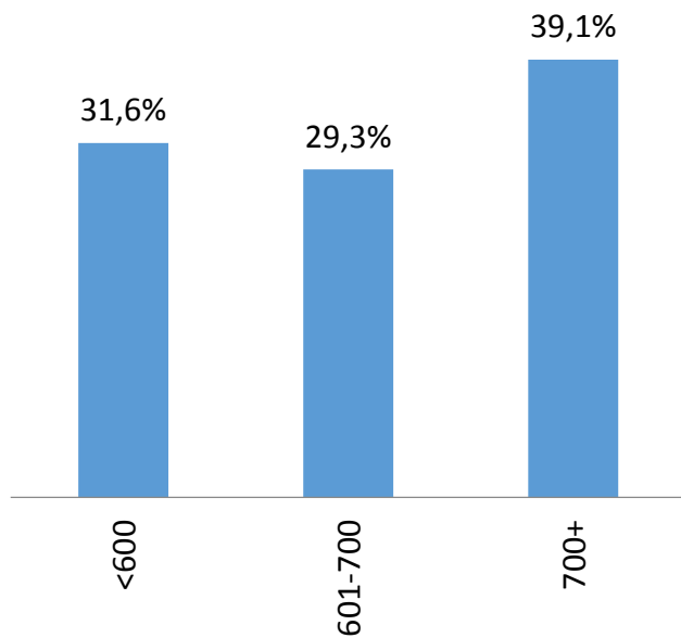
Распределение заявителей на кредиты по диапазонам ПКР
