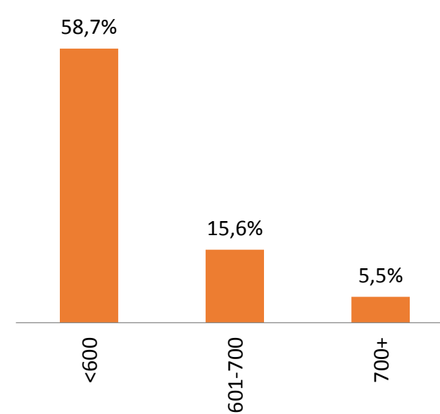
Дефолтность по диапазонам ПКР
